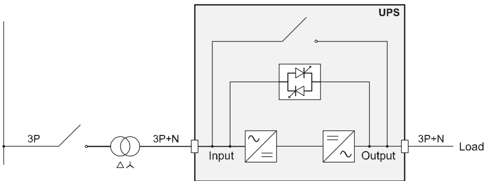
TRI POWER X33 HE mit galvanischer Eingangs-Isolierung
