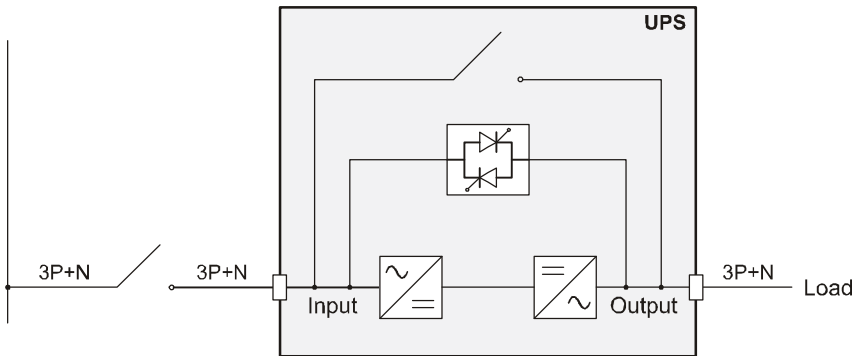
TRI POWER X33 HE ohne Veränderung der Nulleiter-Betriebsart
