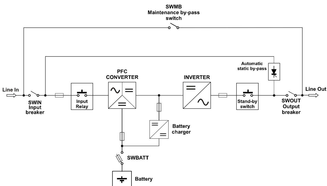
Blockdiagramm der TRI POWER X33 HE
