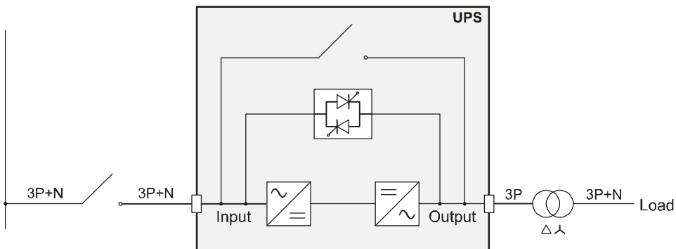
TRI POWER X33 HE mit galvanischer Ausgangs-Isolierung
